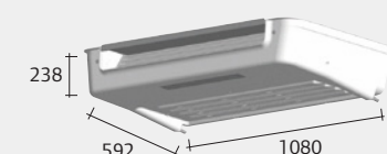
EV-580 Evaporator
