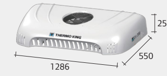
EV-200/EV-300 Condenser(Roof/Nose)
