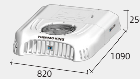
EV-200 Condenser(Roof)
